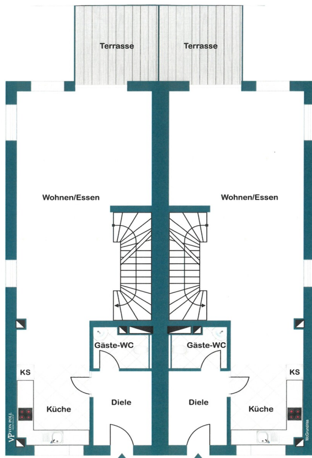
Erdgeschoss
