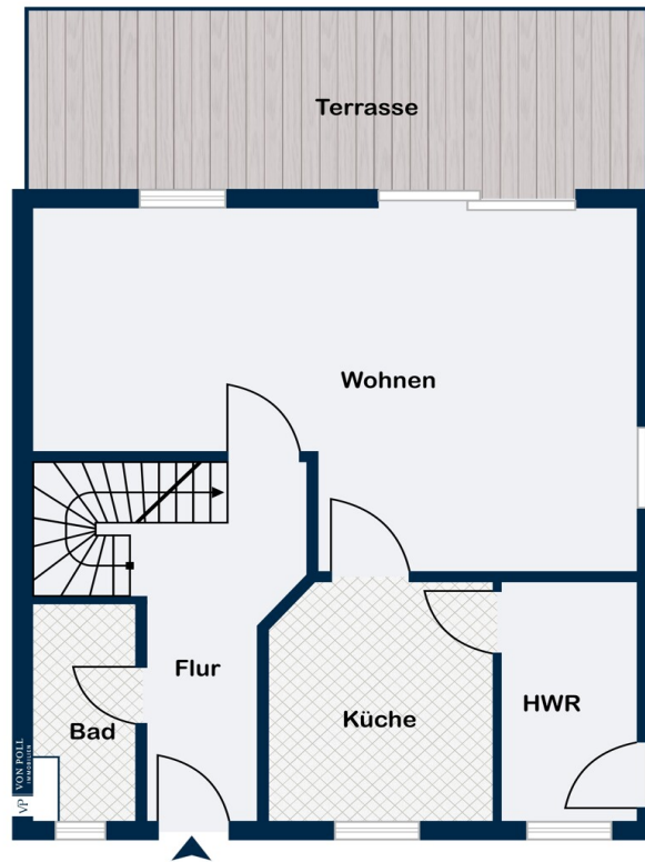
Erdgeschoss
