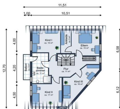
Obergeschoss
