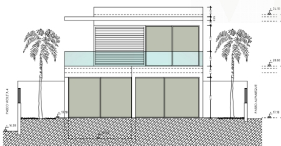
alzado a paseo Violeta 4
