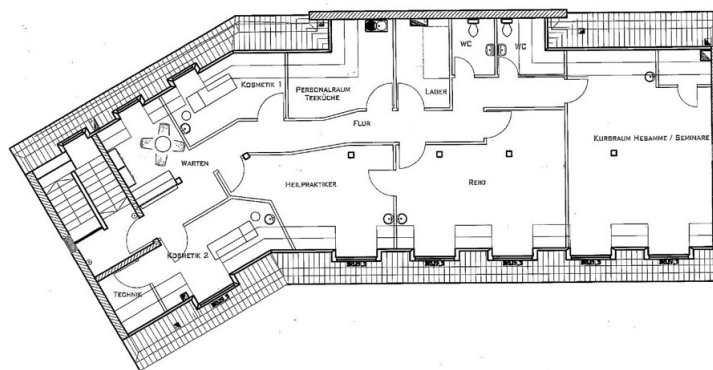
GRUNDRISS 2. OBERGESCHOSS
