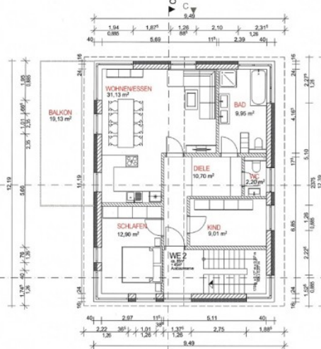
GRUNDRISS OBERGESCHOSS
