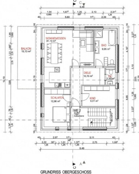
GRUNDRISS OBERGESCHOSS
