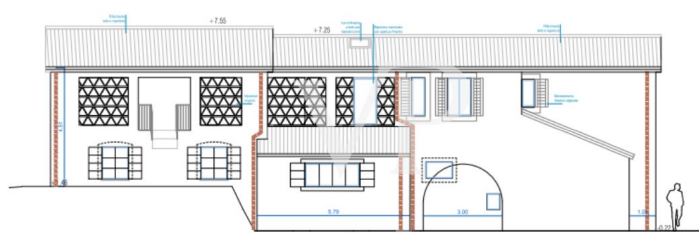
PROSPETTO RETRO
