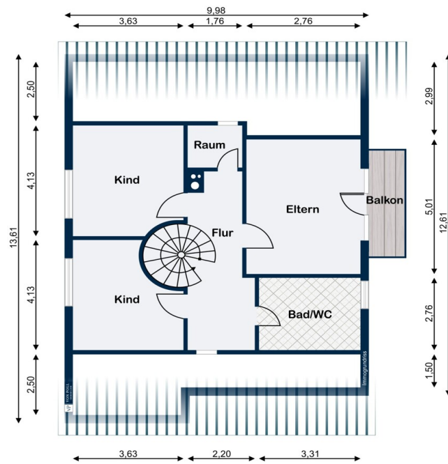
Obergeschoss
