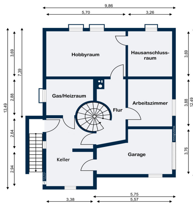
Kellergeschoss
