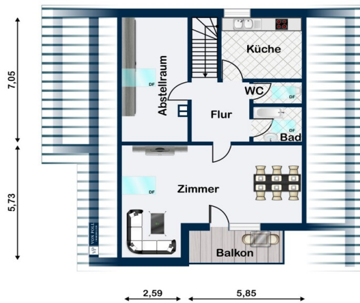
Dachgeschoss
