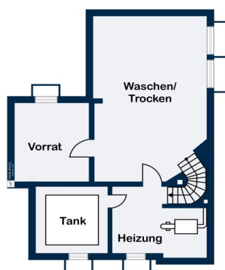
Kellergeschoss
