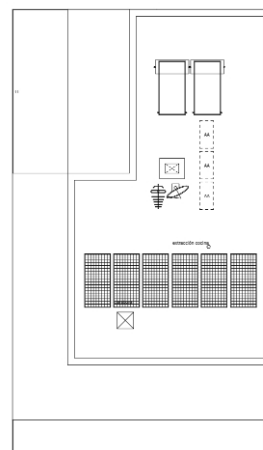
PLANTA CUBIERTA
