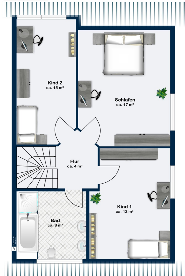
Dachgeschoss
