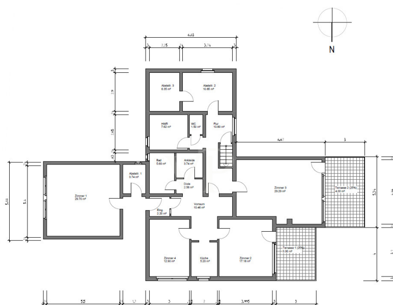
Untergeschoss
