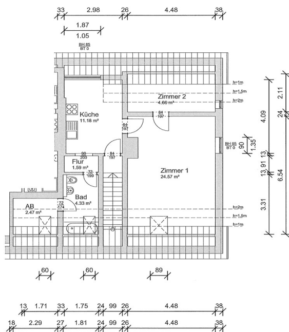
Dachgeschoss: Wohnung 3
